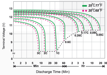
نمودار دشارژ
